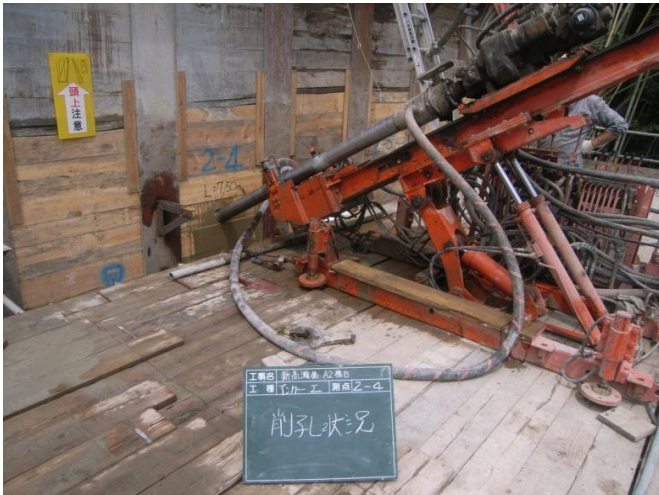
2段目のアンカー工の施工をしています。
